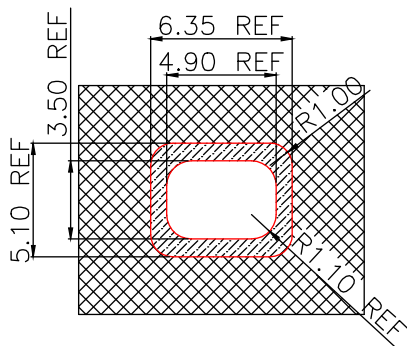
面板开孔参考尺寸
